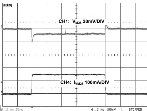
V_{\text{M28}} Load Transient
