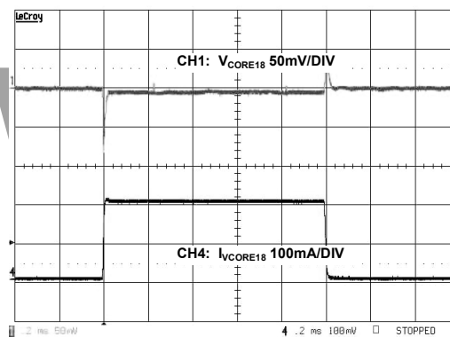
V_{\text{CORE18}} Load Transient
