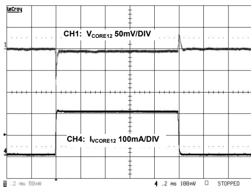
V_{\text{CORE12}} Load Transient
