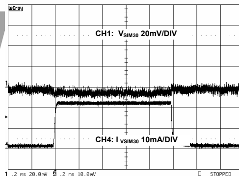
V SIM30 Load Transient
