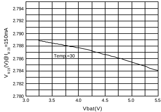
V_{M28} vs. V_{bat}
