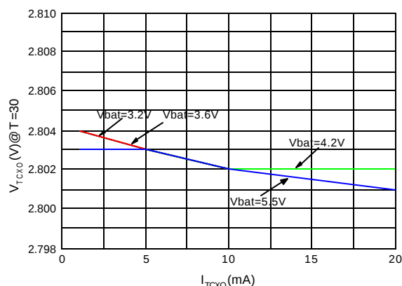
V_{TCXO} vs. I_{TCXO}
