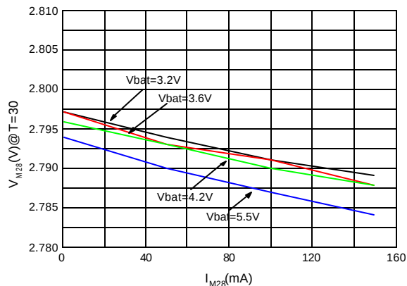
V_{M28} vs. I_{M28}
